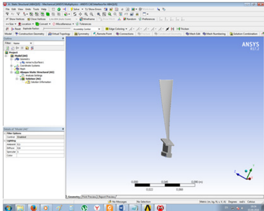
Рисунок 2 - Лопасть последней ступени ГТД
