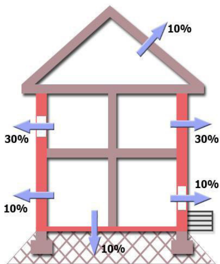
Рис. 3 - Усредненные значения тепловых потерь через ограждающие конструкции здания
