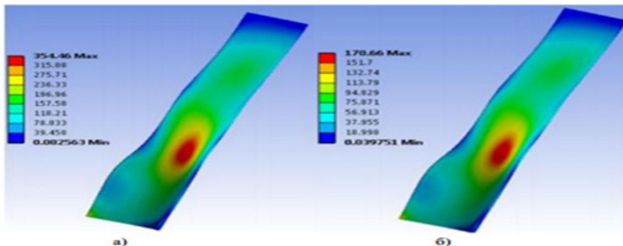
Рисунок 5 - Распределение растягивающих напряжений в (а) титановой Вт-5 и (б) TiC
