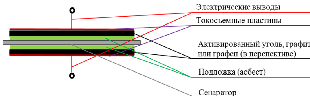
Рисунок 2 – Конструкция ионистора
