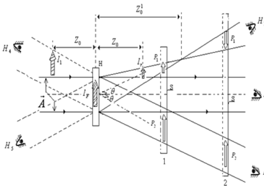
Рисунок 1- Схема освещения голограммы плоской волной \bar{A} . H-голограмма; I_r , I_I и I_f -соответственно действительное, мнимое и сфокусированное изображения объекта; P_1 и P_2 - проекционные изображения объекта; S -экран; 1,2- пространственные положения экрана S .
