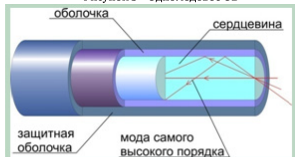
Рисунок 4 – Многомодовое ОВ
