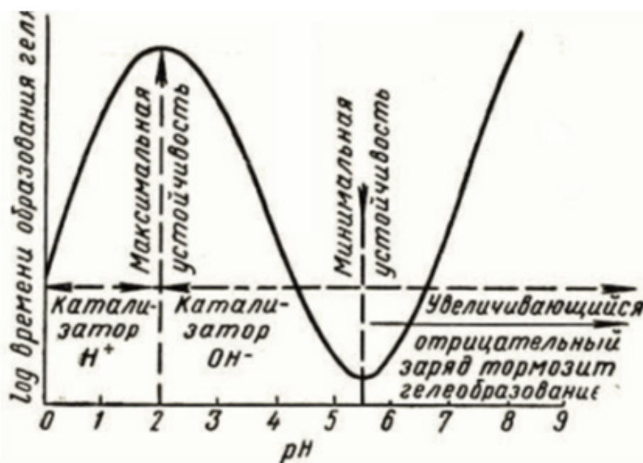
Рисунок 4 - Зависимость устойчивости кремнезольного золя от pH раствора
