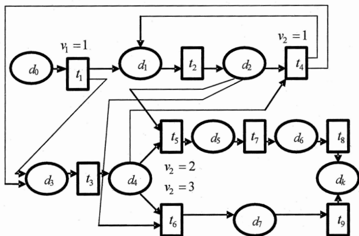
Рис. 3. Сеть Петри как основа графа действий
