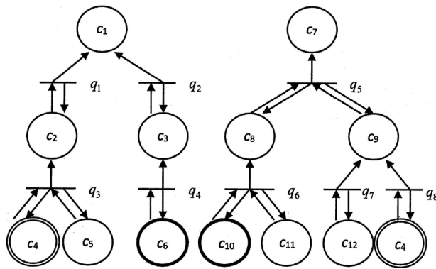
Рис. 1. Пример сети Петри, являющейся основой графа целей
