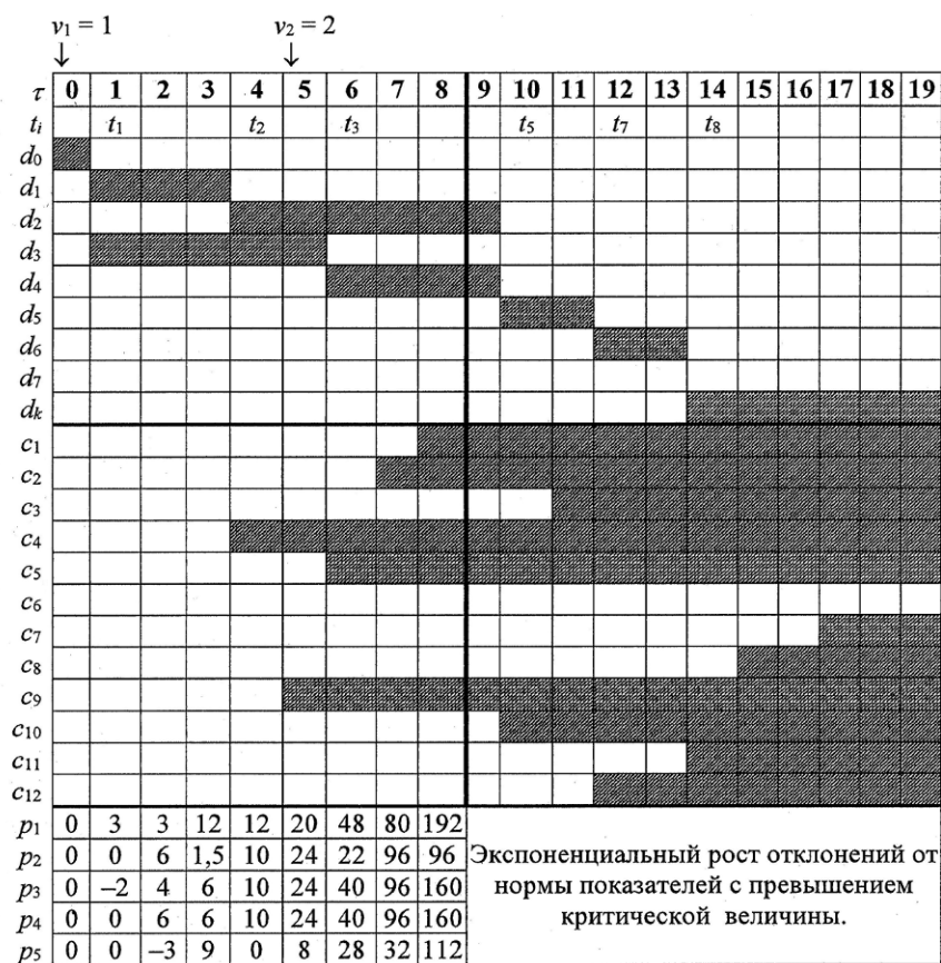
Рис. 4. Итоговая диаграмма моделирования триадной структуры агента
